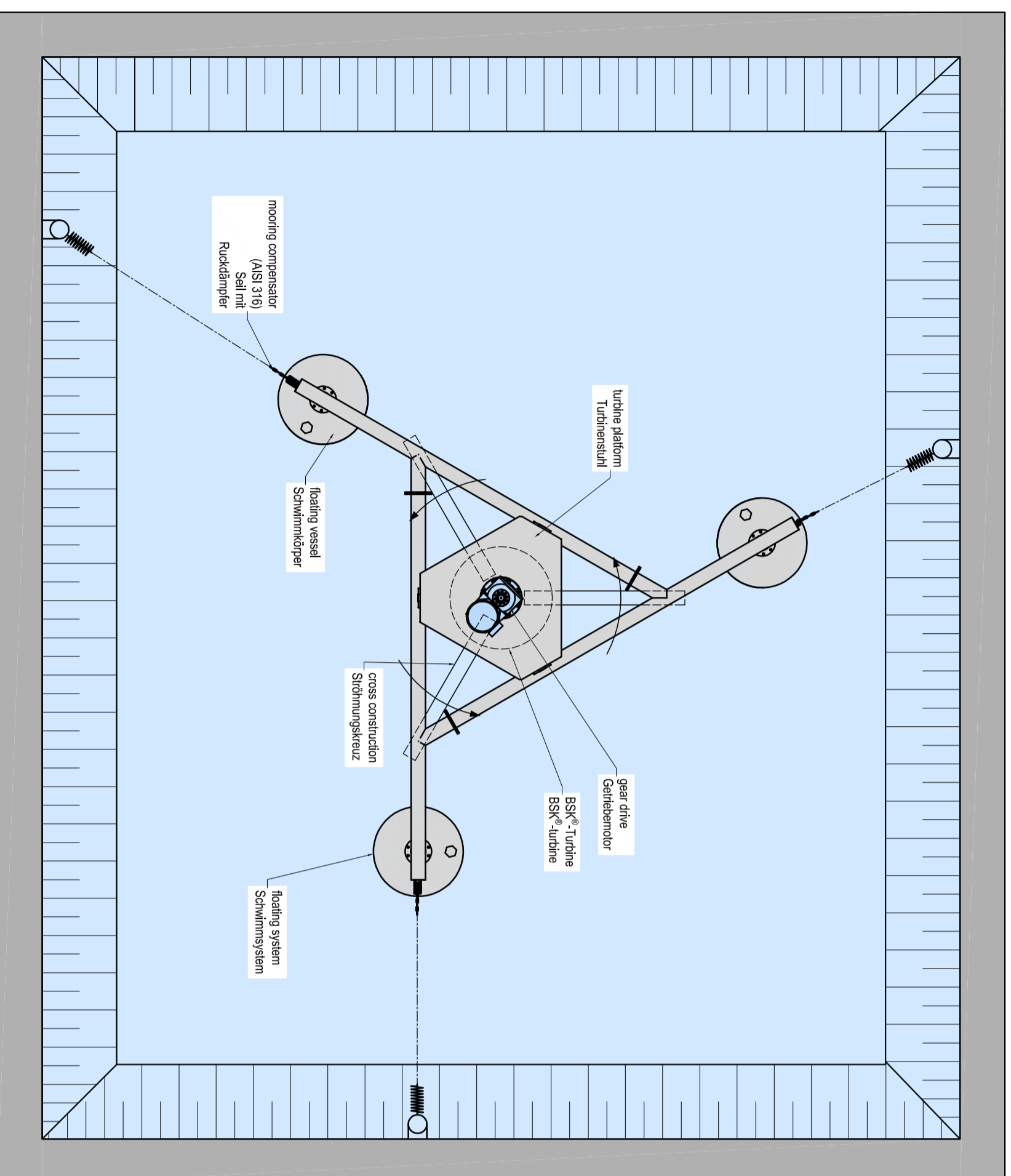
DRAUFSICHT TOP VIEW
